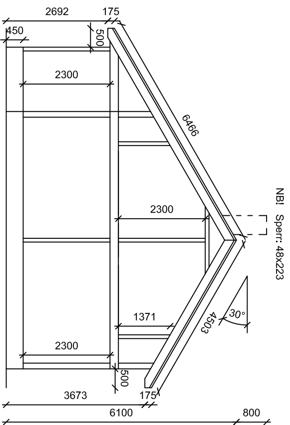
Snitt B - B
