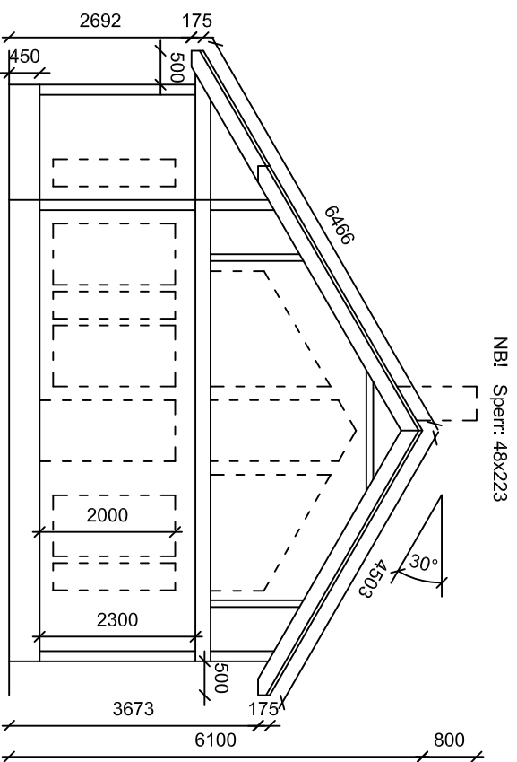
Snitt A - A
