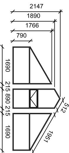
Snitt A - A
