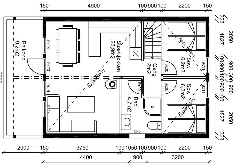
LOFTSPLAN
