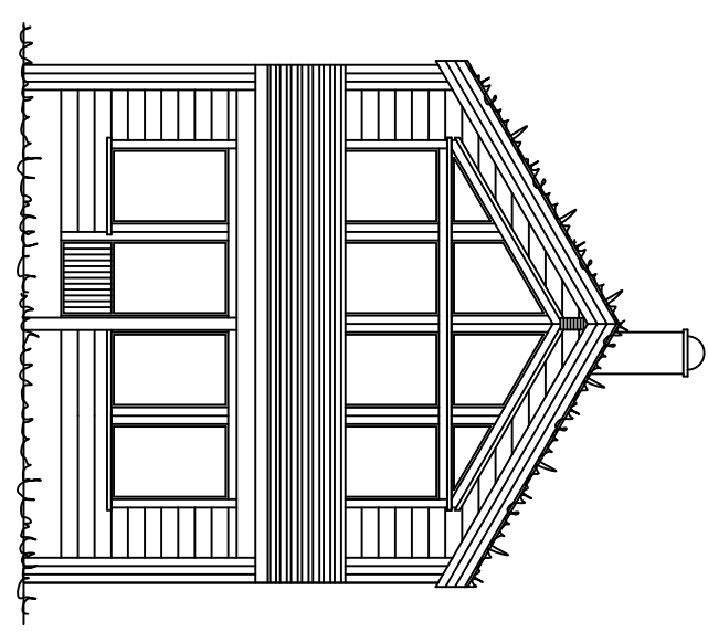
FASADE MOT
